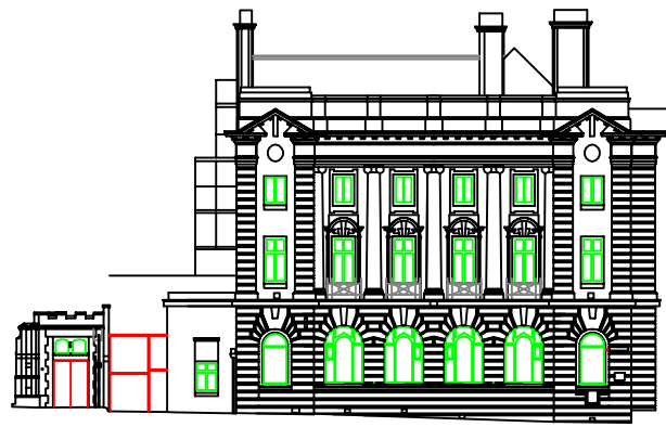
Elevation 5
